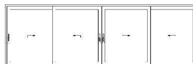
4-teiliges Element mit vier Hebe-Schiebeflügeln
